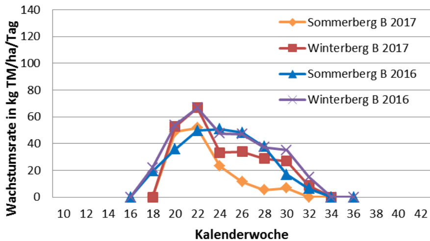
Abb. 3: Mittlere Gras-Wachstumsrate von extensiven Weiden in Bernau (B) in den Kalenderwochen 10 bis 42 der Jahre 2016 und 2017, jeweils am Süd- und am Nordhang.
