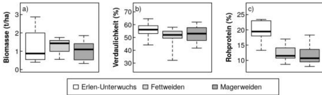
Abb. 2. Stehende Biomasse über 5 cm Schnitthöhe (a), Verdauulichkeit (b) und Rohprotein-Gehalt in der Trockenmasse (c) in drei Vegetationstypen des Beweidungsexperimentes. Der Kasten zeigen den 50% Wertebereich, dicke Linien die Medianwerte und die gestrichelten Linien den gesamten Wertebereich (angepasst aus Zehnder et al. 2016a und 2017).
