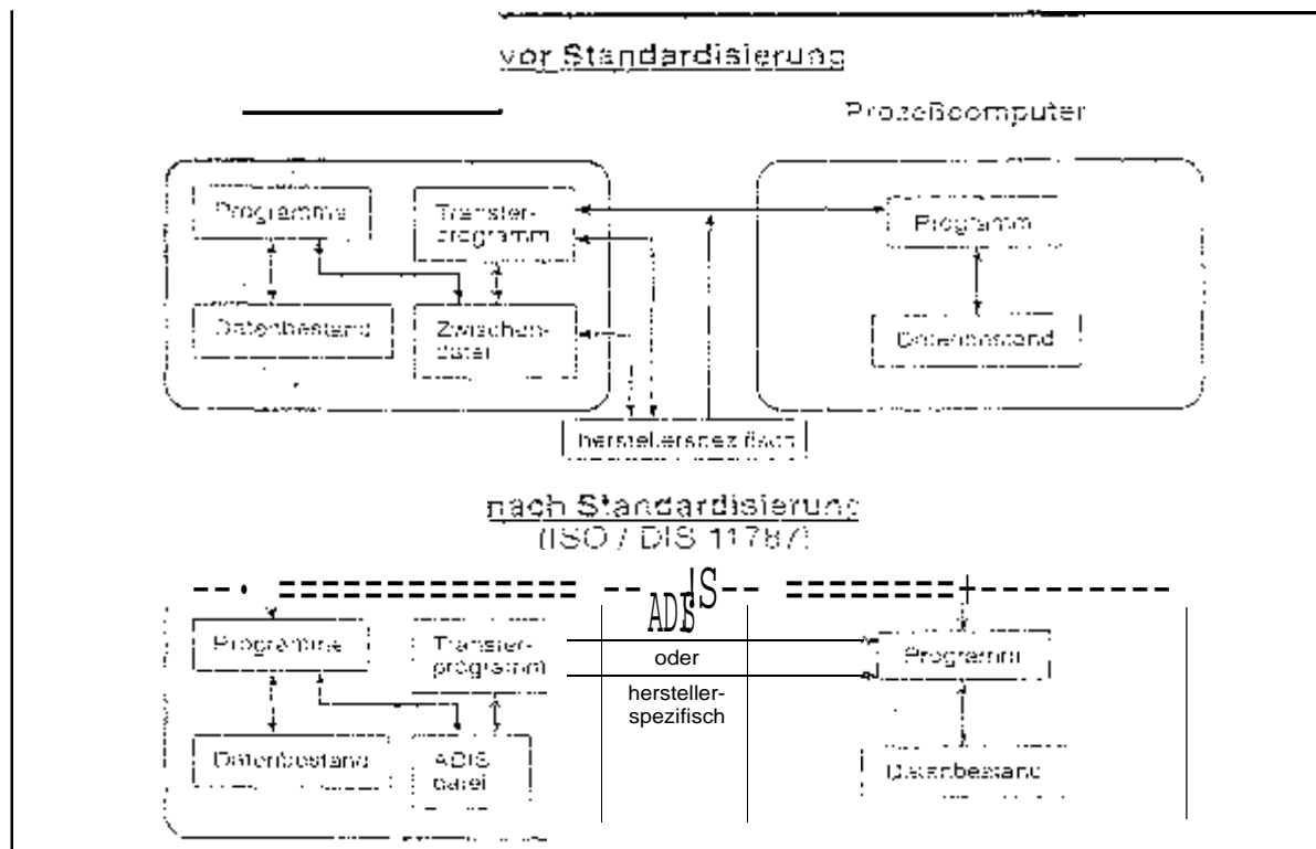
1: Datentransfer zwischen Betriebscomputer und Prozeßrechner
