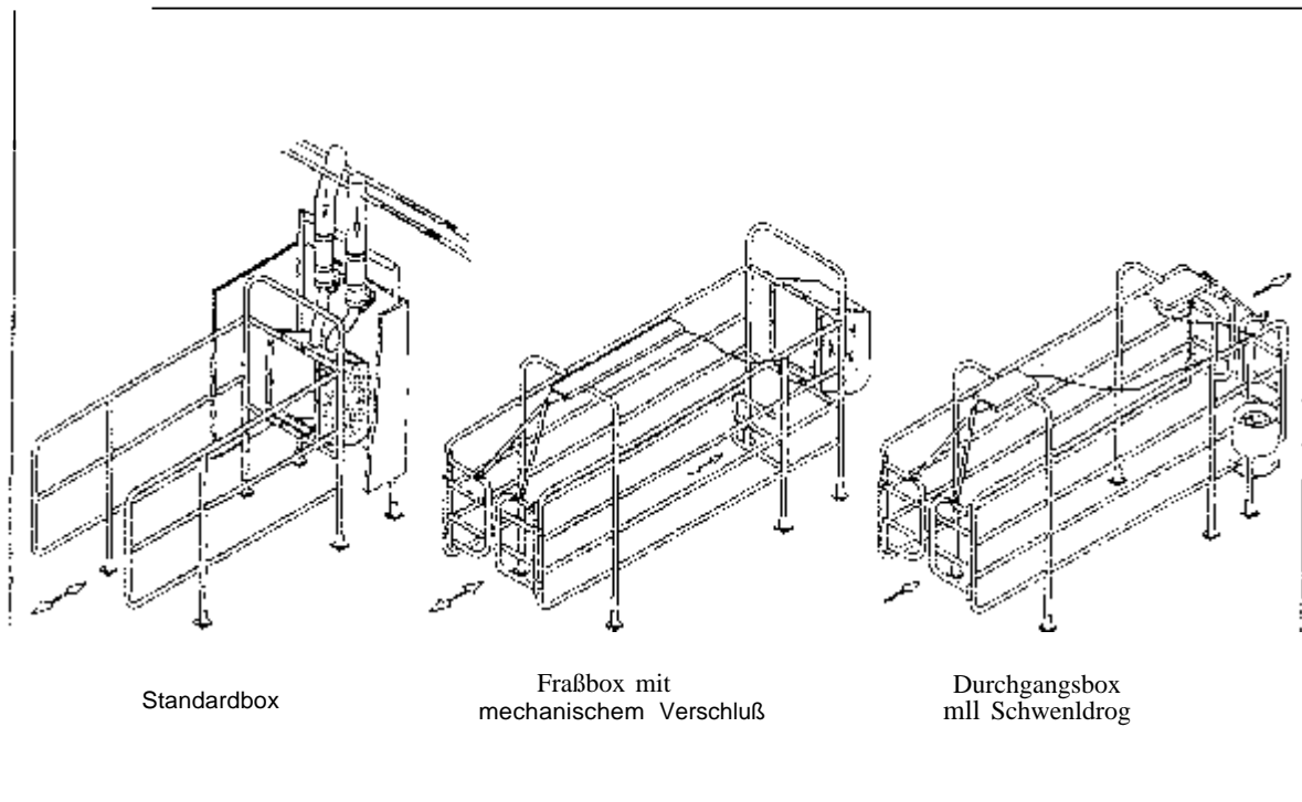
Abb. 7: Freißstandformen für Kraftfutterabruflanlagen
