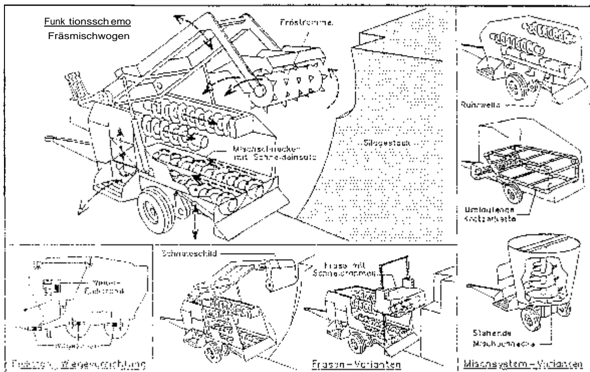
Abb. 3: Bauarten von Fräsmischwagen
