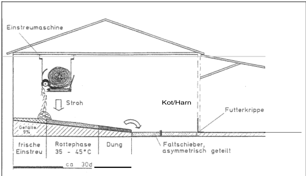
2: Funktionsprinzip des Tretmiststalles
