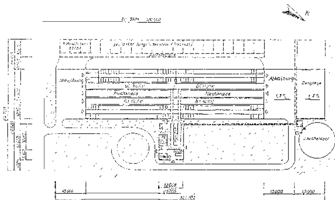
Grundriß zum Milchviehstall Gladigau (Kaltstall mit Festmist für 240 Milchkuhe)
