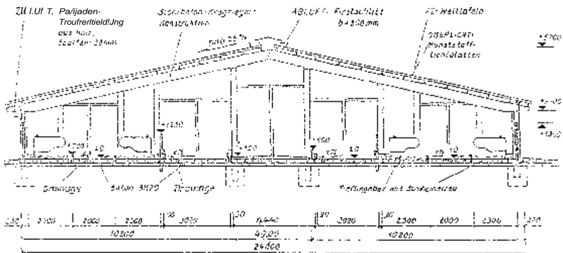
Abb. 2. Schnitt zu Milchviehstall Gladigau (Kaltstall Festmist Milchkuhe)
