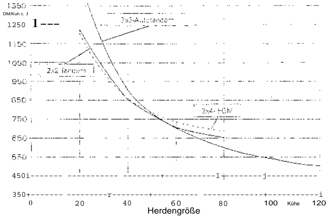
Kosten der Arbeitserledigung verschiedener Melkstände in Abhängigkeit von der Bestandesgröße -I- (1/6 Trockensteher, Lohnansatz 15 DM, ohne Kosten für Milchkühlung)
