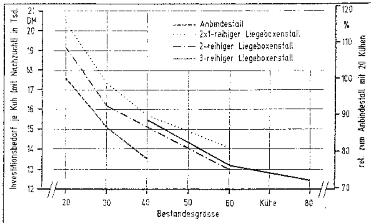
Investitionsbedarf für verschiedene Stallformen
