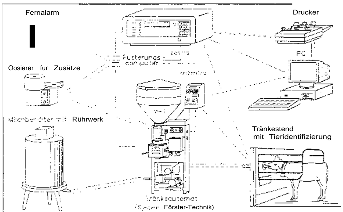
Abb. 6 Funktionsschema rechnergesteuerter Tränkeautomaten für die Kälberhaltung (Pulver- oder Kombiautomat)
