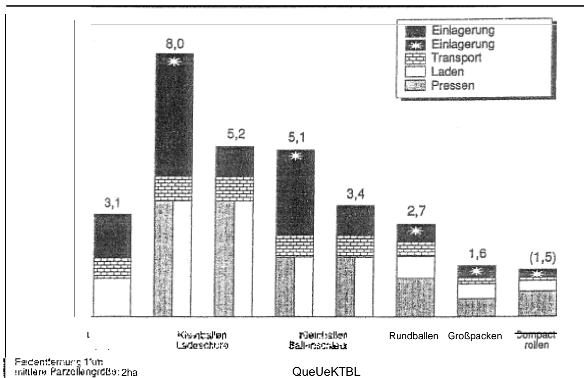
Abb. 3 Arbeitszeitbedarf der Strohbergeverfahren (50 dt Stroh je ha; Quelle KTBL)
