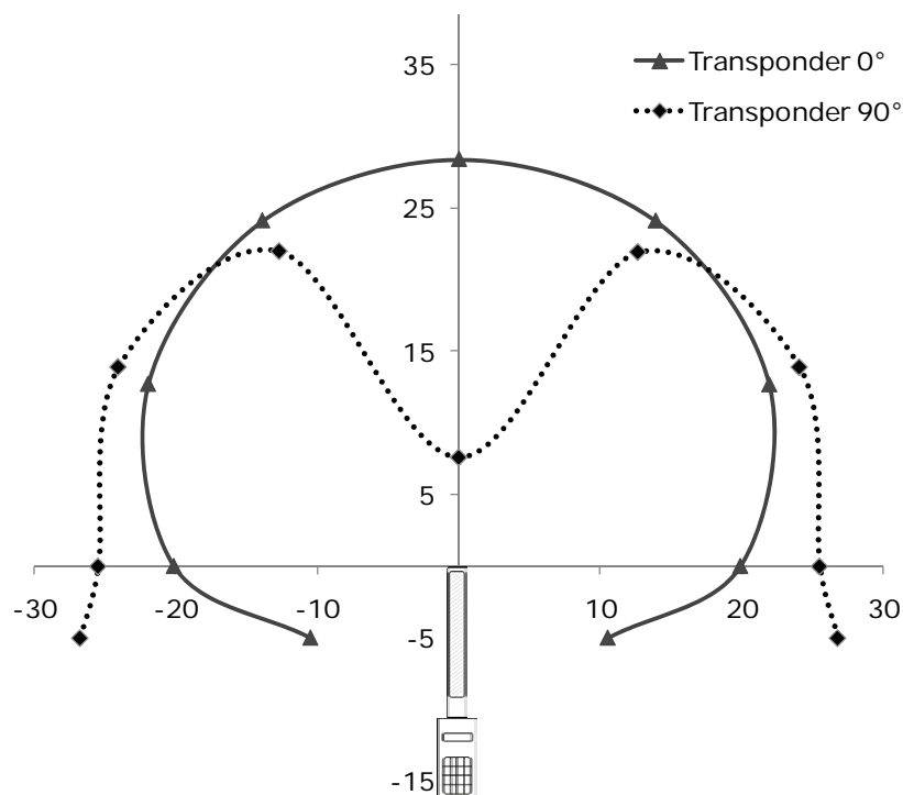
Abb. 24: Schematischer Lesebereich [cm] für ein Lesegerät
