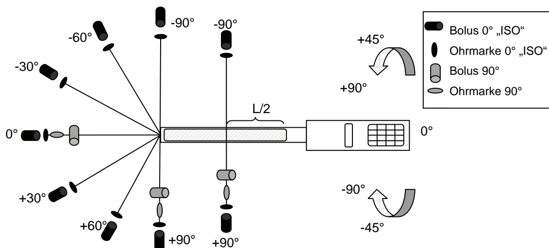
Abb. 6: Messaufbau für die Reichweitenmessung unter Laborbedingungen
