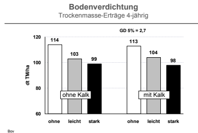
Abb. 1: In den ersten 4 Versuchsjahren wurden in den verdichteten Parzellen deutlich geringerer Erträge gemessen als in den unverdichteten.
