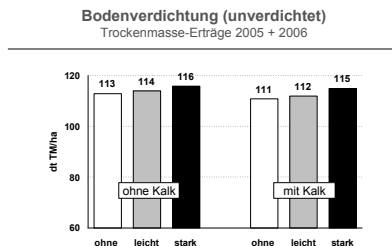
Abb 2: Auswirkung der 4-jährigen Bodenverdichtung.
