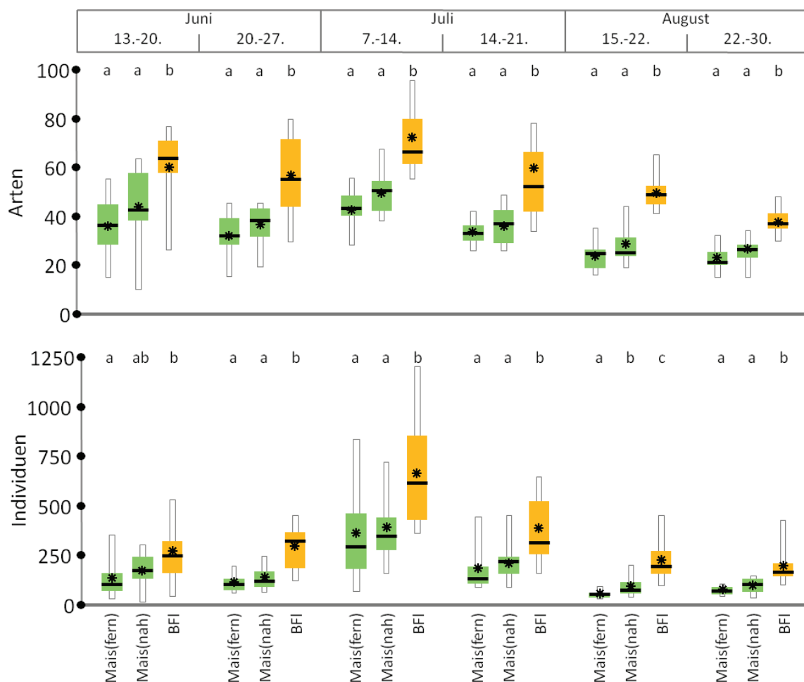
Abb. 19: Artenreichtum (oben) und Abundanz (unten) bei Insekten und Spinnentieren in den 6 Fangperioden 2011, BFI = Blühfläche, Mais(nah) = blühflächennaher Maisacker, Mais(fern) = blühflächenferner Maisacker, n = 13 Standorte á 3 Fallen, Friedman-Test und nachgeschaltet Wilcoxon-Test für jede Fangperiode, unterschiedliche Buchstaben (a, b) geben signifikante Unterschiede an.
