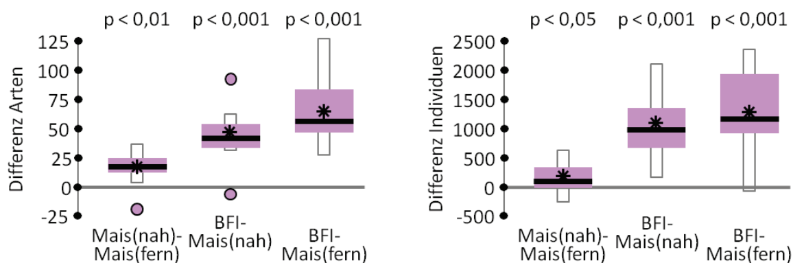
Abb. 20: Arthropoden (Insekten und Spinnentiere), Differenz Arten(reichtum) (links) bzw. Abundanz (Individuen) (rechts), n = 13 Standorte á 3 Fallen, Wilcoxon-Test.
