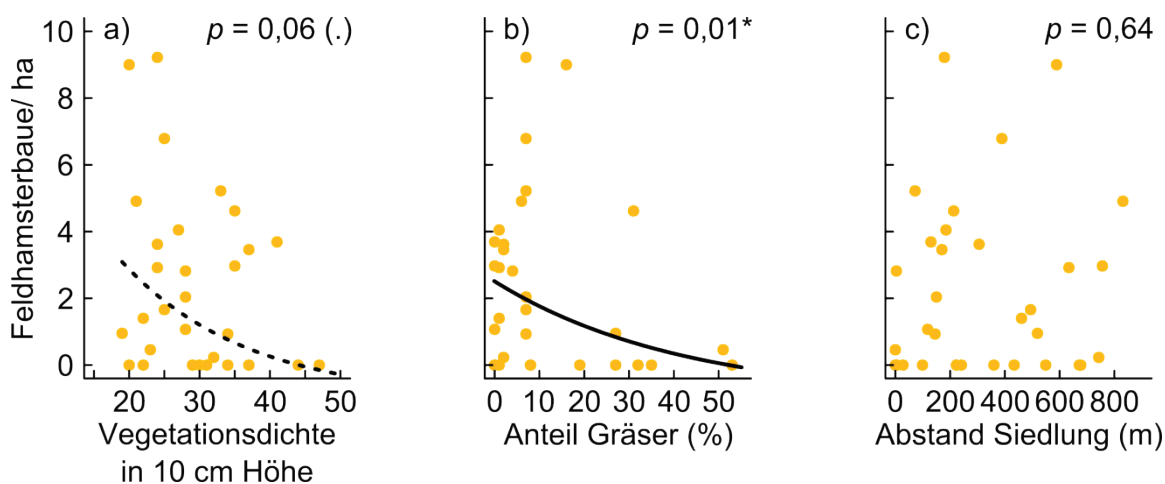
Abb. 39: Ergebnisse der linearen Regressionen für die Feldhamsterdichte in Abhängigkeit von a) der Vegetationsdichte, b) dem Anteil an Gräser und c) dem Abstand zu einer Siedlung.
