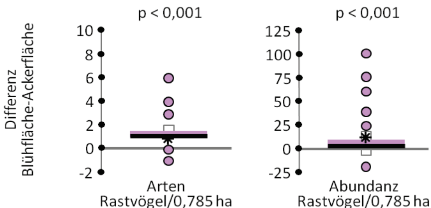
Abb. 31: Rastvögel: Gesamtartenreichtum (Artensumme) und Gesamtabundanz (Individuensumme), zwei Begehungen, dargestellt als Differenzen der n = 40 Paare (jeweils Blühfläche minus Acker), Wilcoxon-Test, siehe (Tab. 25), zur Darstellung siehe WAGNER & VOLZ (2014), Skalierung der Y-Achse beachten.
