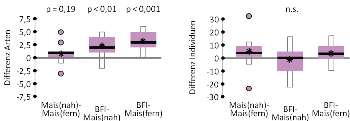
Abb. 21: Arthropoden (Insekten und Spinnentiere) Rote Liste Bayern-Arten, Differenz Arten(reichtum) (links) bzw. Abundanz (Individuen) (rechts), BFI = Blühfläche, Mais(nah) = blühflächennahes Maisfeld, Mais(fern) = blühflächenfernes Maisfeld, n = 13 Standorte á 3 Fallen, n.s. = vorgeschalteter Friedman-Test nicht signifikant, Wilcoxon-Test.
