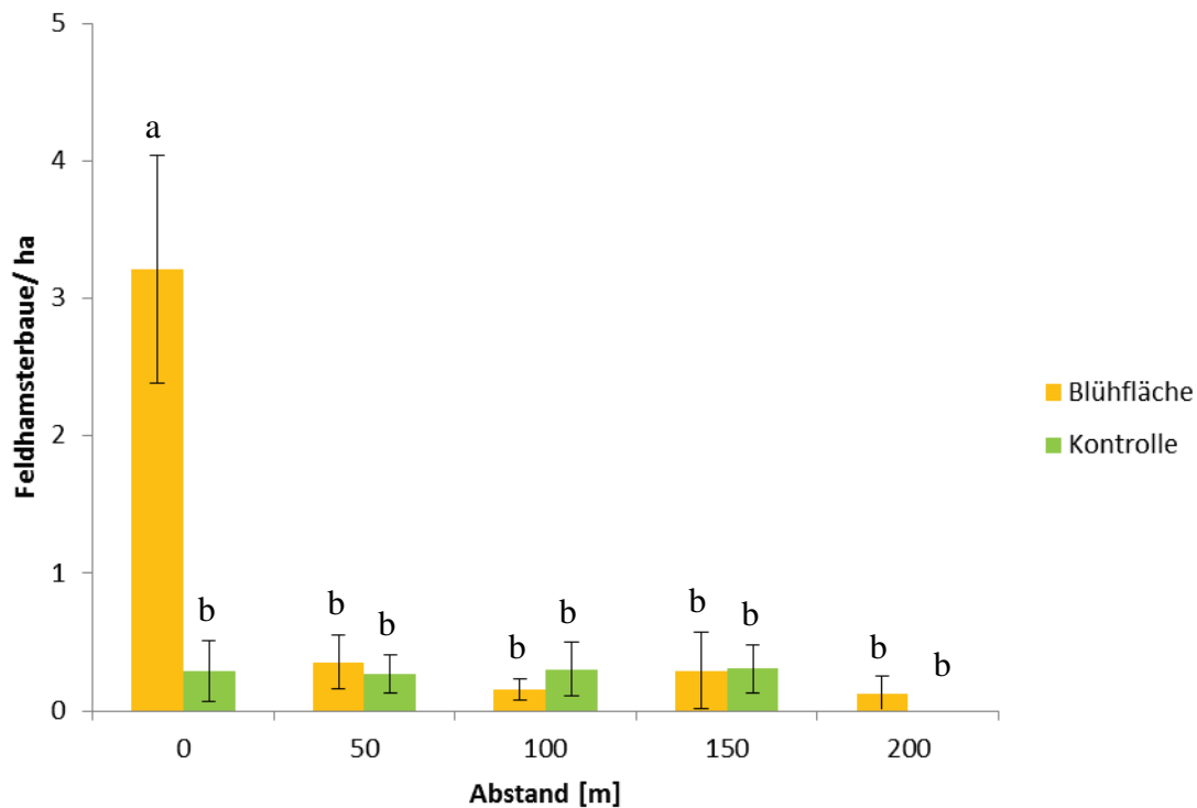
Abb. 38: Ergebnisse des TukeyHSD-post-hoc-Vergleichs für die Feldhamsterdichte (Mittelwert \pm SE, n = 14 ) in Abhängigkeit von Flächentyp und Abstand. Unterschiedliche Buchstaben geben statistisch signifikante Unterschiede zwischen den unterschiedlichen Faktorebenen an.
