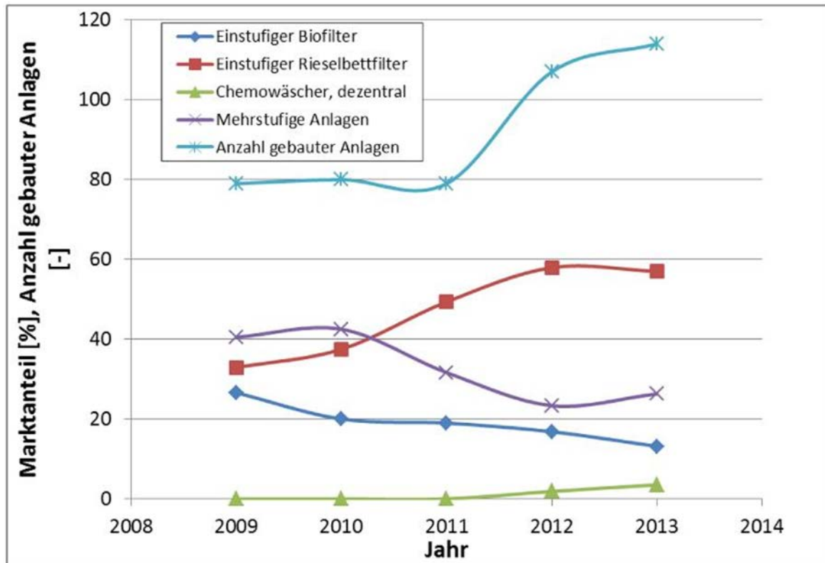
Abb. 3: Entwicklung der Anzahl gebauter Abluftreinigungsanlagen in der deutschen Schweinehaltung (Quelle: UBA 2016)
