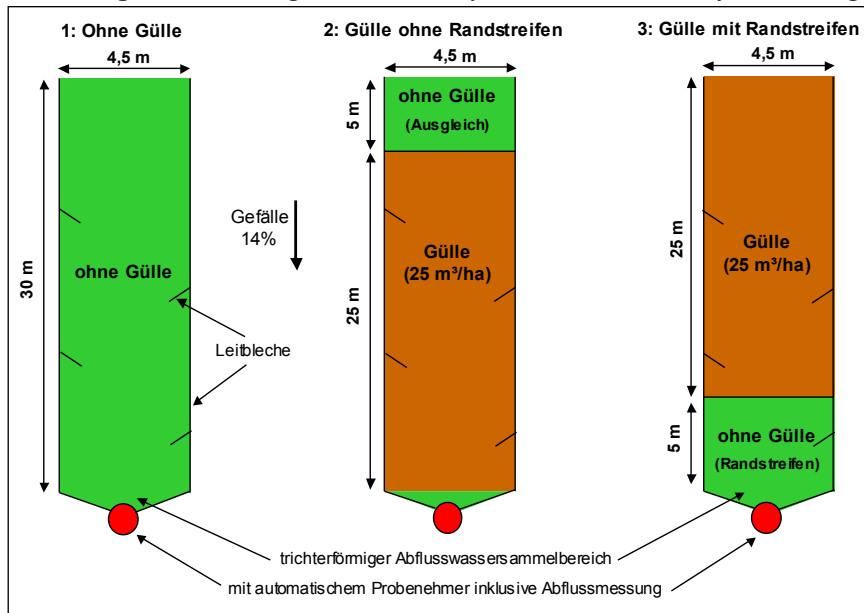
Abbildung 1: Darstellung von Versuchsaufbau, Varianten und Abflussmessung
