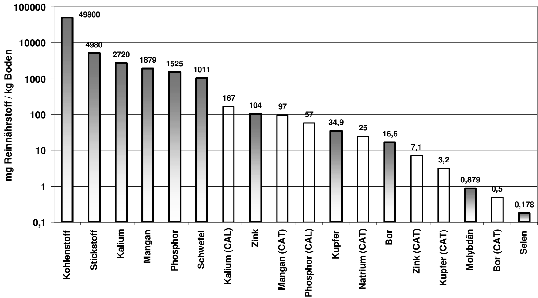
Abbildung 1: Durchschnittliche Nährstoffgehalte (n = 30) von Grünlandböden in 0-10 cm Tiefe
