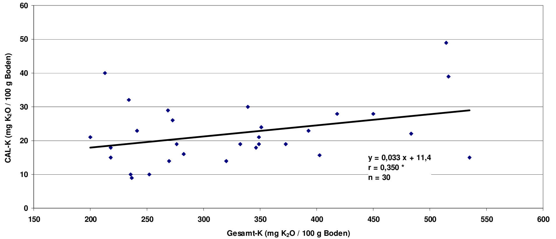
Abbildung 6: Beziehung zwischen Gesamt-Kaligehalt und pflanzenverfügbarem Kali
