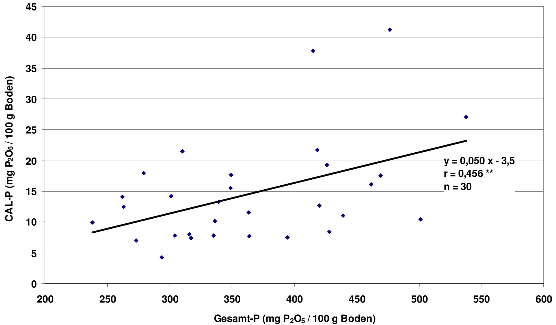
Abbildung 5: Beziehung zwischen Gesamt-Phosphatgehalt und pflanzenverfügbarem Phosphat
