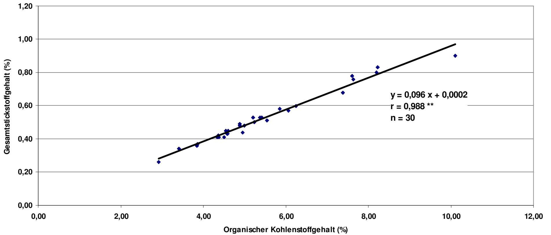
Abbildung 3: Beziehung zwischen Kohlenstoff- und Stickstoffgehalt unter Grünland in 0-10 cm Tiefe
