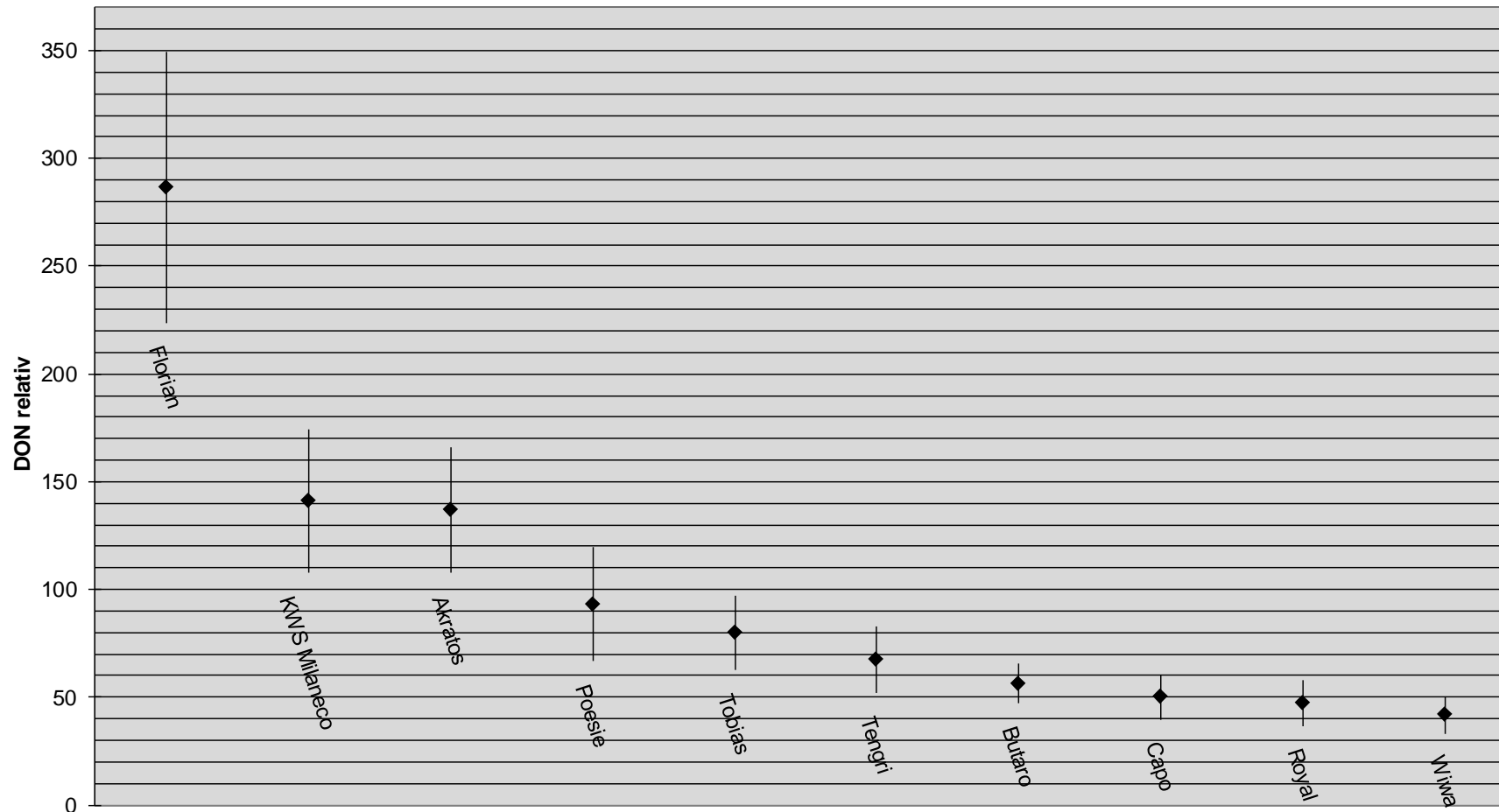
Relativwerte von DON Winterweizen 2018-2014 mit 90%-Konfidenzintervallen
