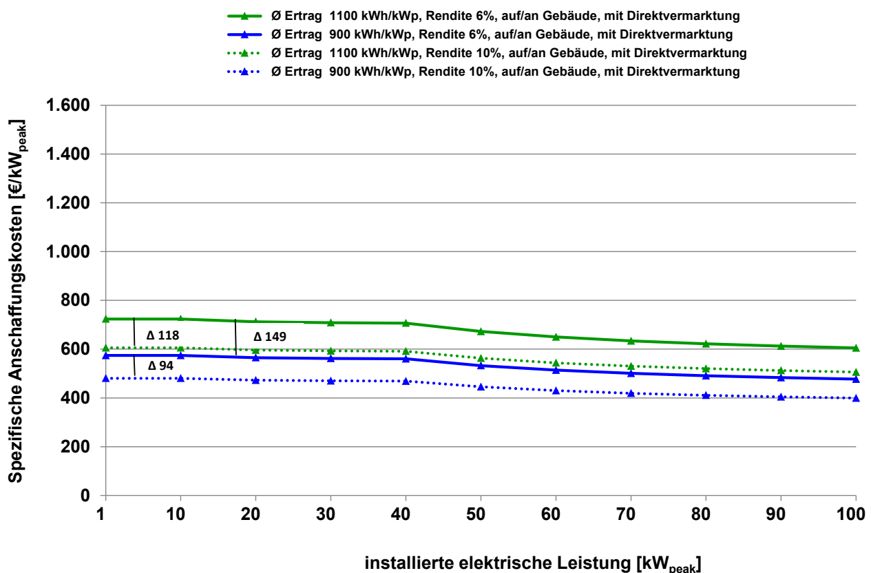
Abbildung 1: „Höchstens tragbare“ Anschaffungskosten einer PV-Dachanlage bis 100 kW p im September 2021
