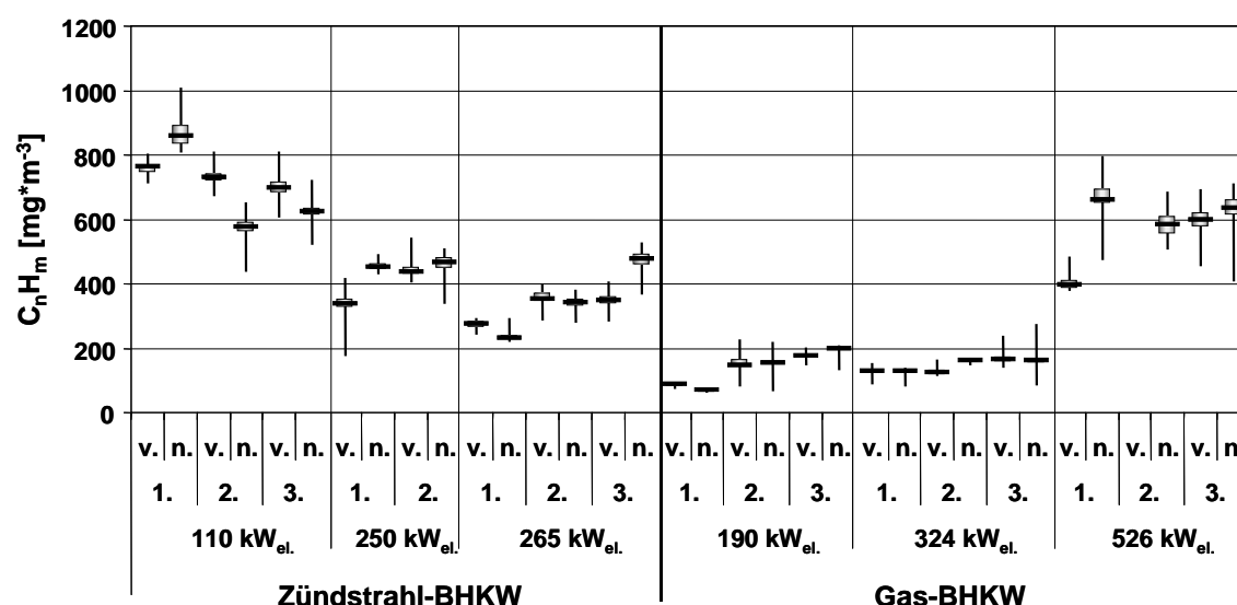
Abb. 25: Box-Plot der C n H m -Gehalte im Abgas aller drei Messreihen der untersuchten BHKW vor (v.) und nach (n.) einer Wartung
