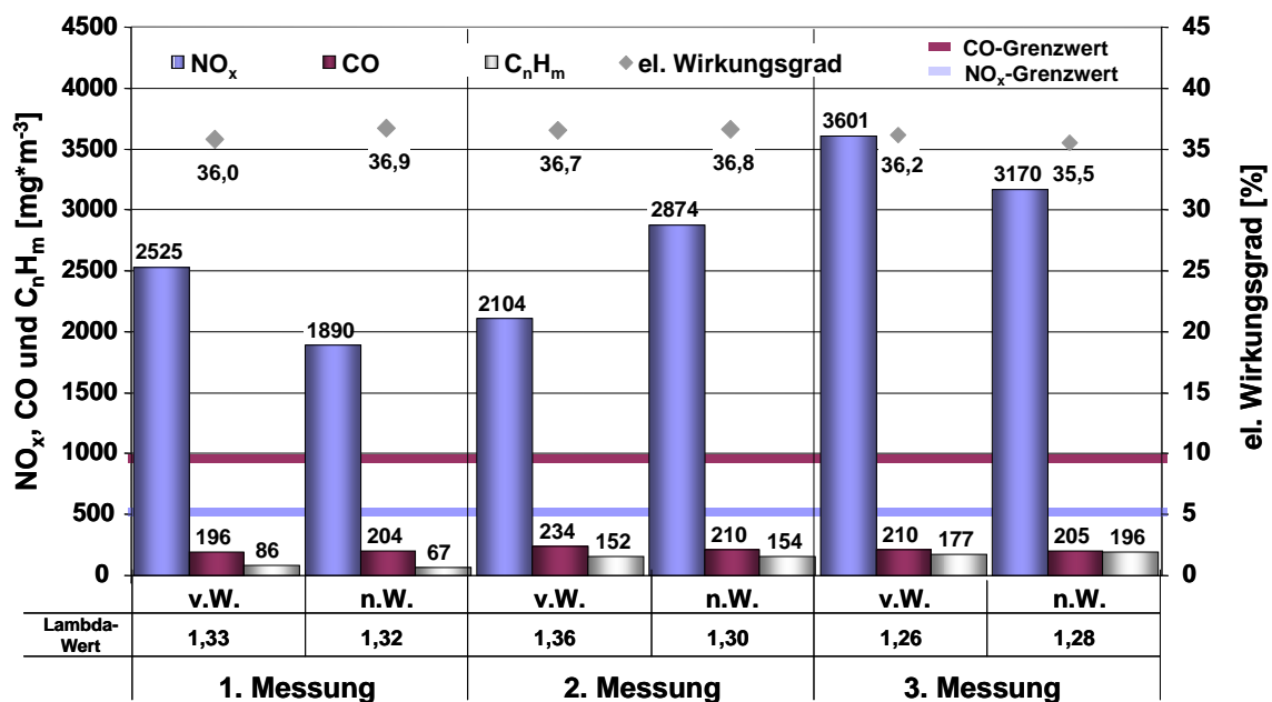
Abb. 19: Abgaskonzentrationen und elektrische Wirkungsgrade des 190 kW el. Gas-BHKW (v.W.= vor Wartung; n.W.= nach Wartung)
