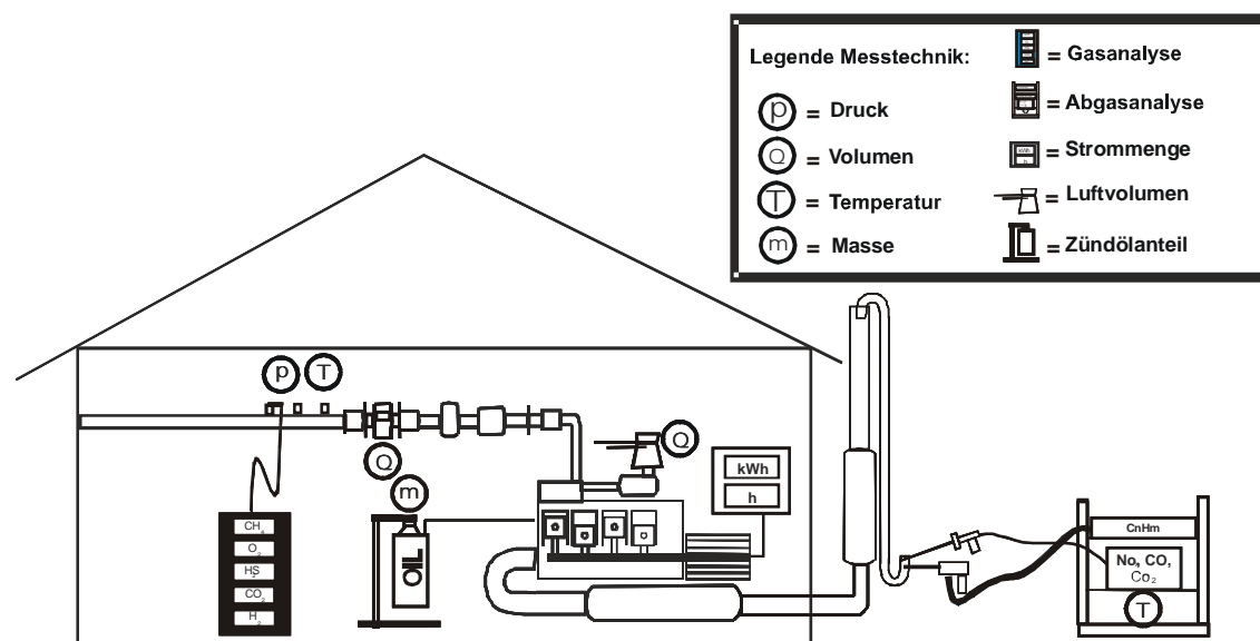
Abb. 7: Aufbau für die kontinuierliche Messung des Leistungs- und Emissionsverhaltens eines BHKW unter Praxisbedingungen
