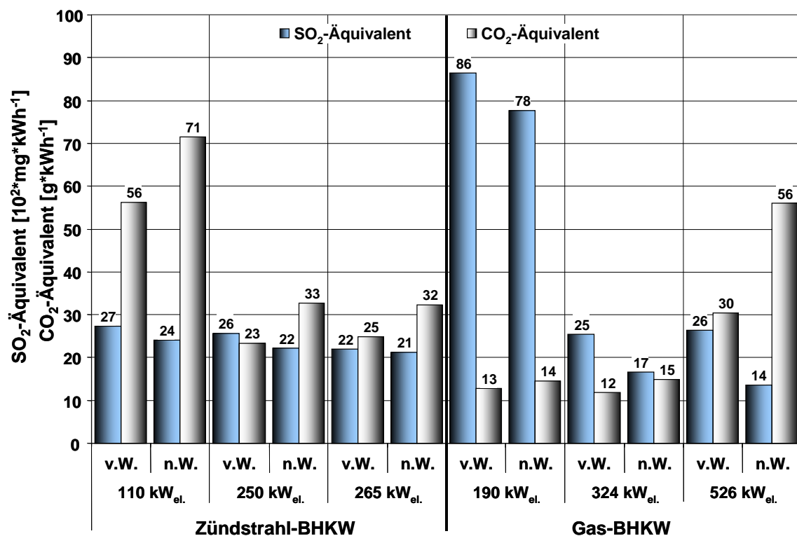
Abb. 31: CO 2 - und SO 2 -Äquivalentemissionen der untersuchten BHKW
