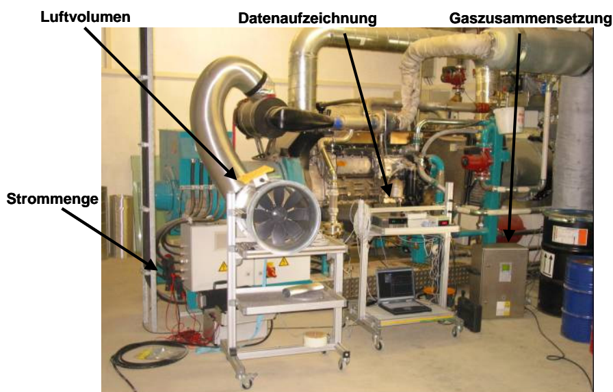
Abb. 8: Messgeräteaufbau am BHKW in der Praxis
