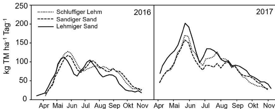
Abb. 1: Tägliche Wachstumsraten ( \text{kg TM ha}^{-1} \text{ Tag}^{-1} ) der intensiv beprobten und konventionell bewirtschafteten Flächen in 2016 und 2017 bei einer N-Düngung von 280 \text{ kg N ha}^{-1} \text{ Jahr}^{-1} .
