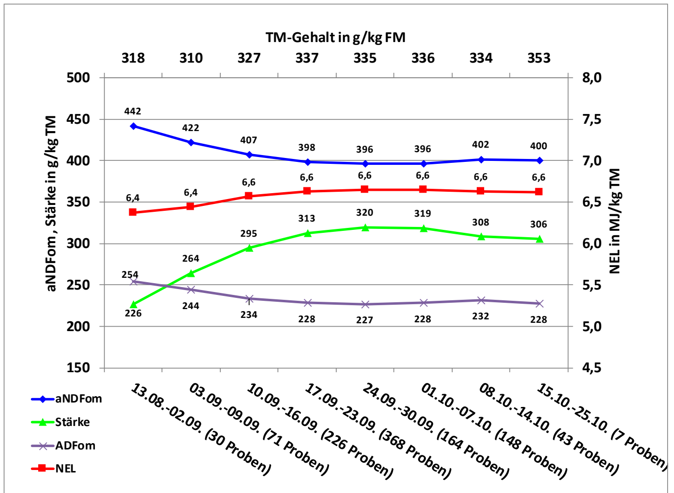
Abb.: Verlauf von aNDF om , ADF om , Stärke und Energie in Abhängigkeit vom Erntetermin
