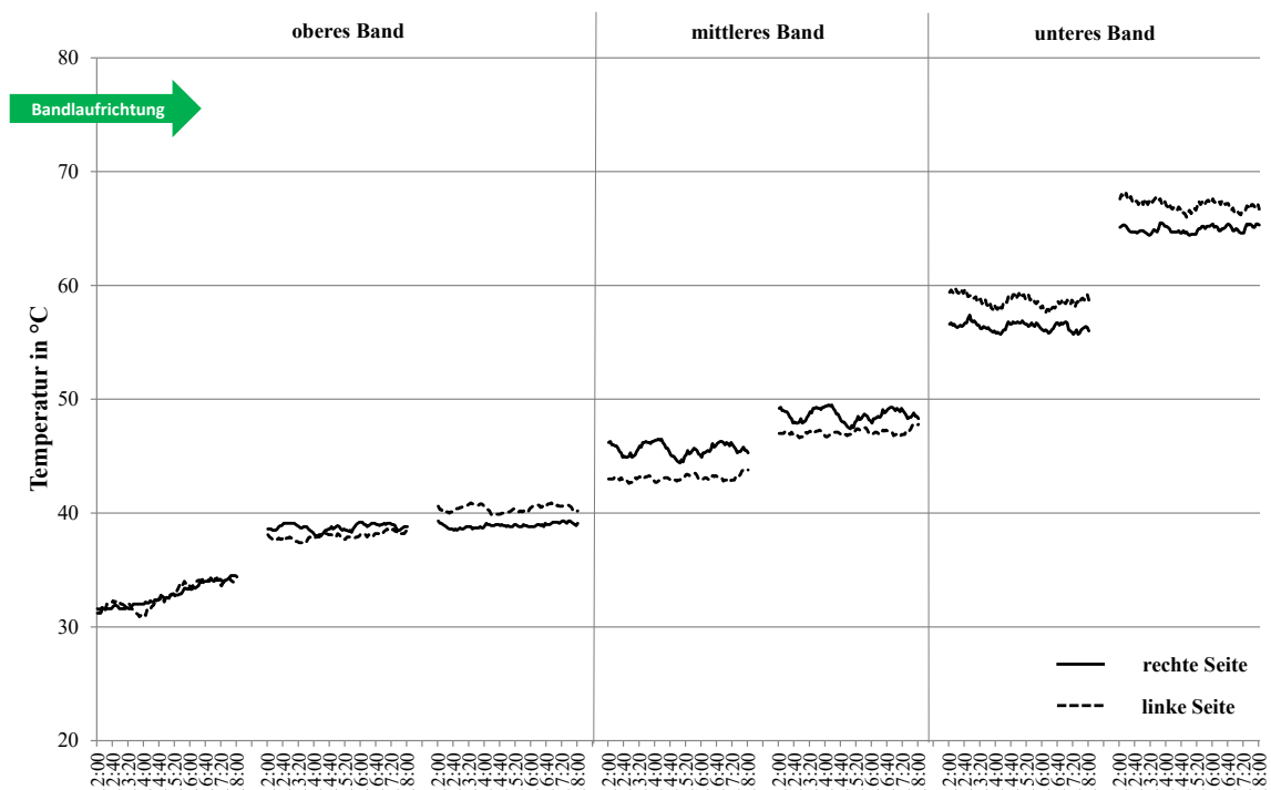
Abb. 31: Gleichmäßiger Temperaturanstieg der durchströmenden Trocknungsluft über allen Trocknungsbändern
