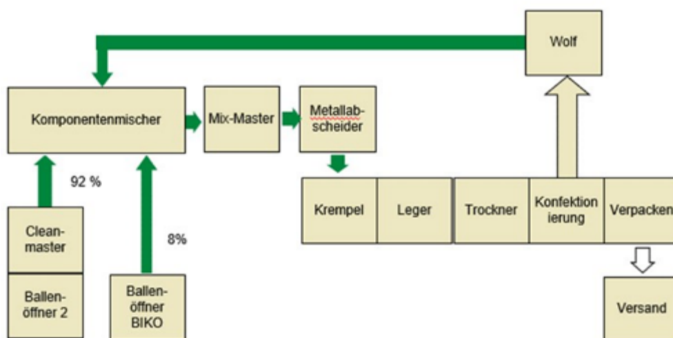
Abb. 23: Prozessfolge der Dämmstofffertigung bei der Firma HempFlax Building Solution GmbH in Nördlingen, Darstellung des Unternehmens
