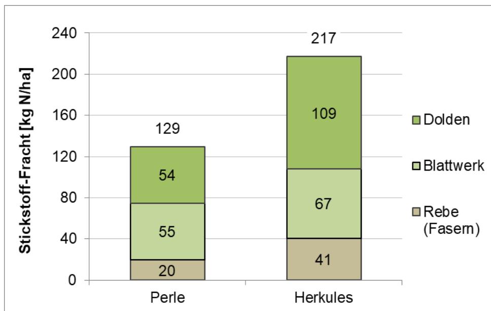
Abb. 29: Stickstofffracht zum Zeitpunkt der Ernte gegliedert in je 3 Fraktionen der Hopfensorten Perle und Herkules, 2023, leichter Standort (LS)
